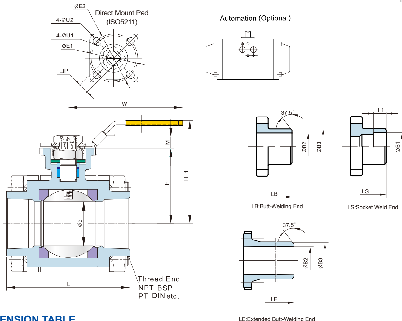
ANSI 2000 WOG DIMENSION TABLE
